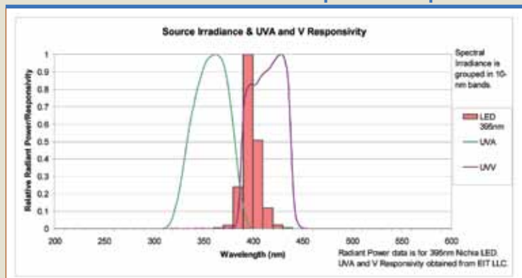
Spectral output of a 395 nm LED source and EIT UV-A and EIT UV-V radiometer spectral response
